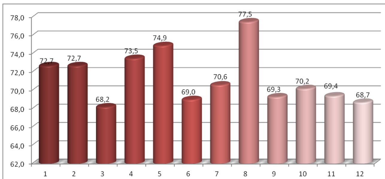
55 pav. Maksimalaus triukšmo pasiskirstymas matavimo vietose dienos metu (7-19 val.). Ribinis dydis 70 dBA.
