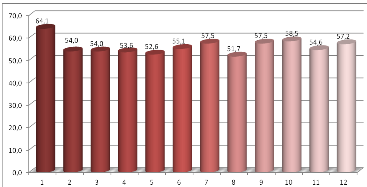
65 pav. Maksimalaus triukšmo pasiskirstymas matavimo vietose vakaro metu (19-22val.). Ribinis dydis 65 dBA.
